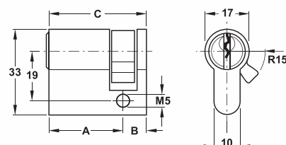
普通齿锁芯
