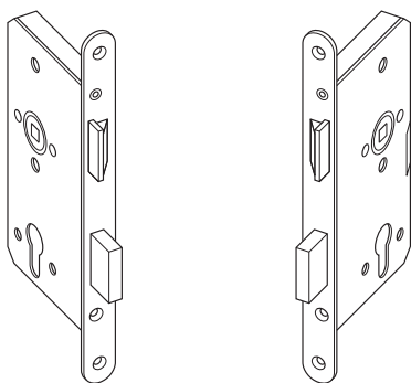
DIN 左式锁体/LH (面对斜舌直边，斜舌 在左侧即为左式锁体)
