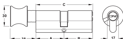
电脑齿锁芯
