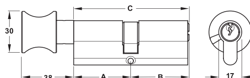
电脑齿锁芯
