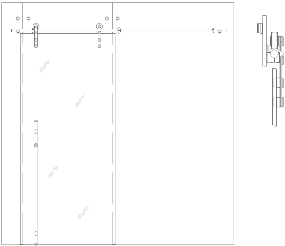
玻璃门侧装件
