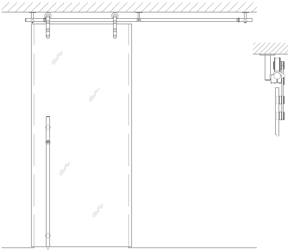
吊装件
