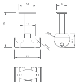
双移门屋顶支撑
