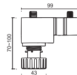
可调脚卡扣 (配铝合金或塑料踢脚板) Adjustable feet clip
